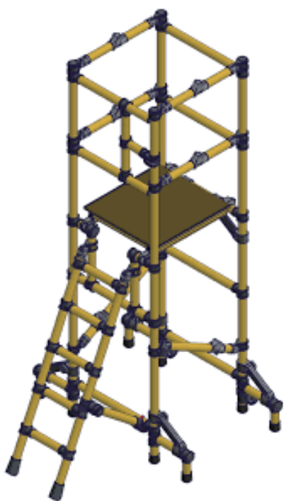
平台由 0.95M 至 1.5M高 載重 150kg 符合PAS250 最大工作平台高度小於2.5m
